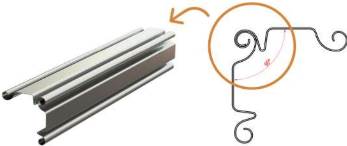
Perfil Meia Cana Liso
